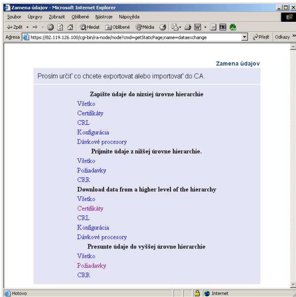
Obr. 43: Presuvanie požiadaviek a certifikátov medzi CA a RA
