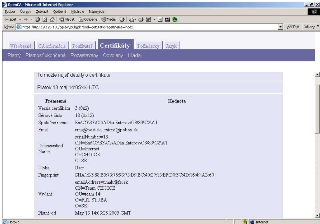
Obr. 40: Údaje o certifikáte
