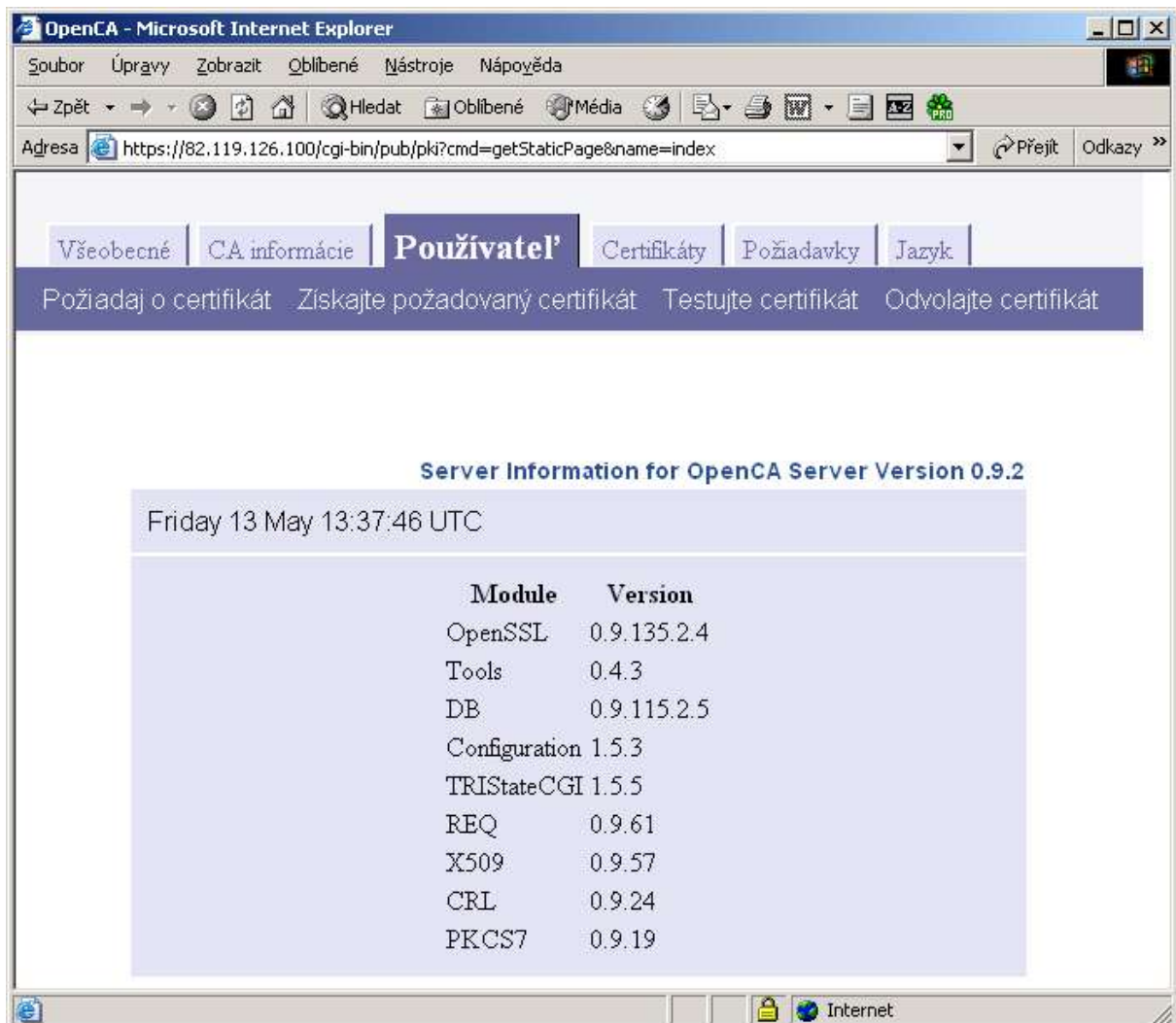
Obr. 36: Verjná časť RA
