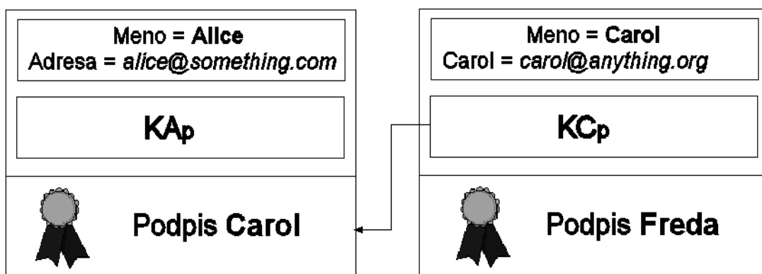
Obr. 8: Reťazenie certifikátov
