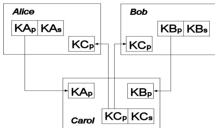
Obr. 21: Sprostredkovateľ - počiatočná výmena kľúčov
