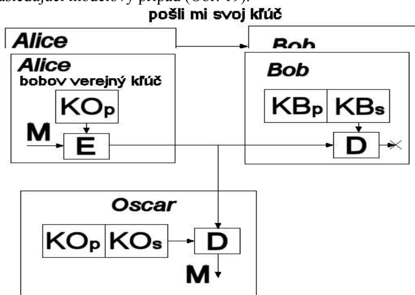
Obr. 20: Záměna kľúčov II.
