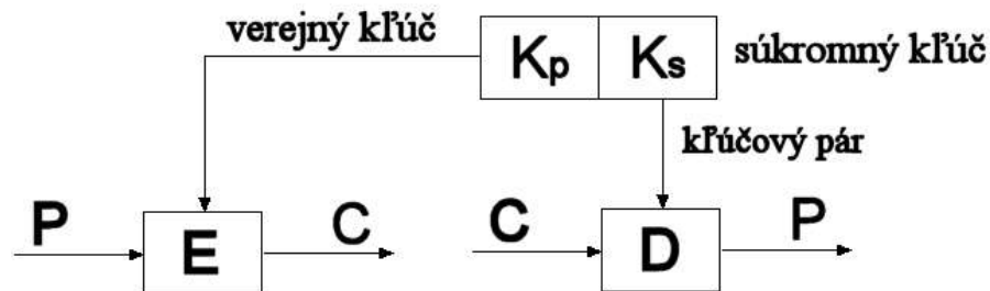
Obr. 24: Asymetrická šifra
