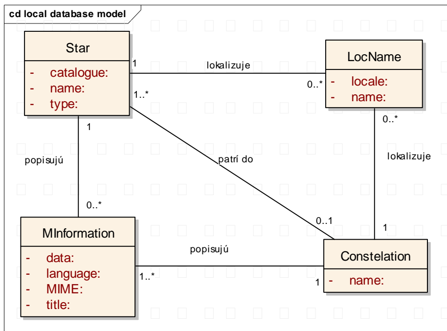
Obr. 10 Logický dátový model pre lokálnu databázu údajov
