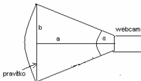
Obr. 5 Spôsob merania uhla pohľadu kamery
