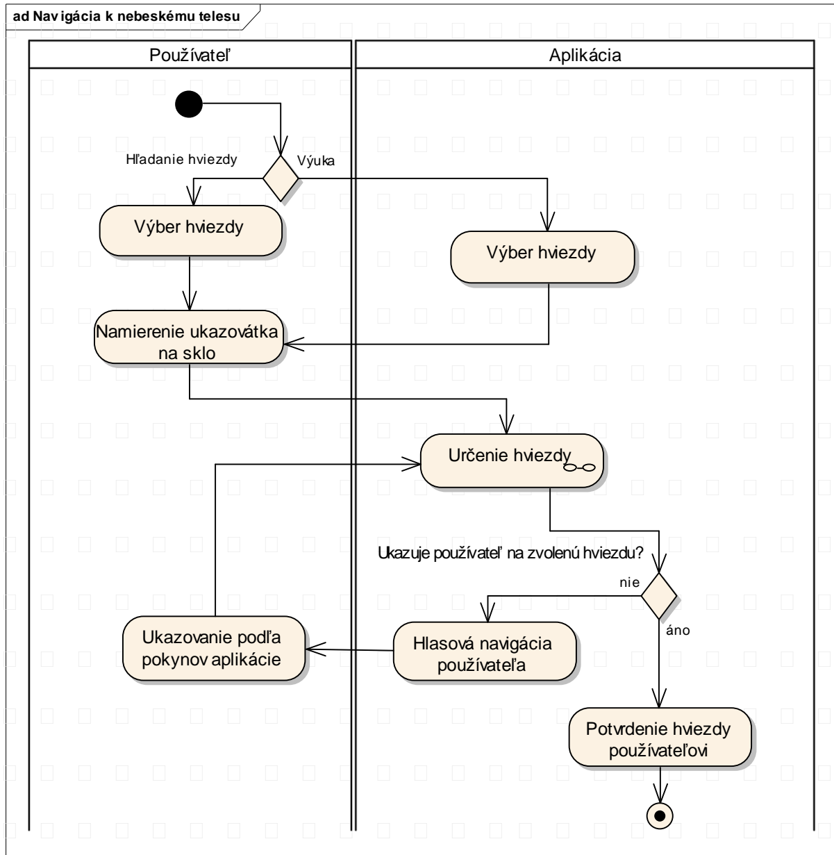
Obr. 8 Diagram aktivít pre prípad použitia navigácia k nebeskému telesu
