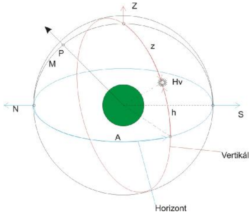
Obr. 2 Nebeská sféra
