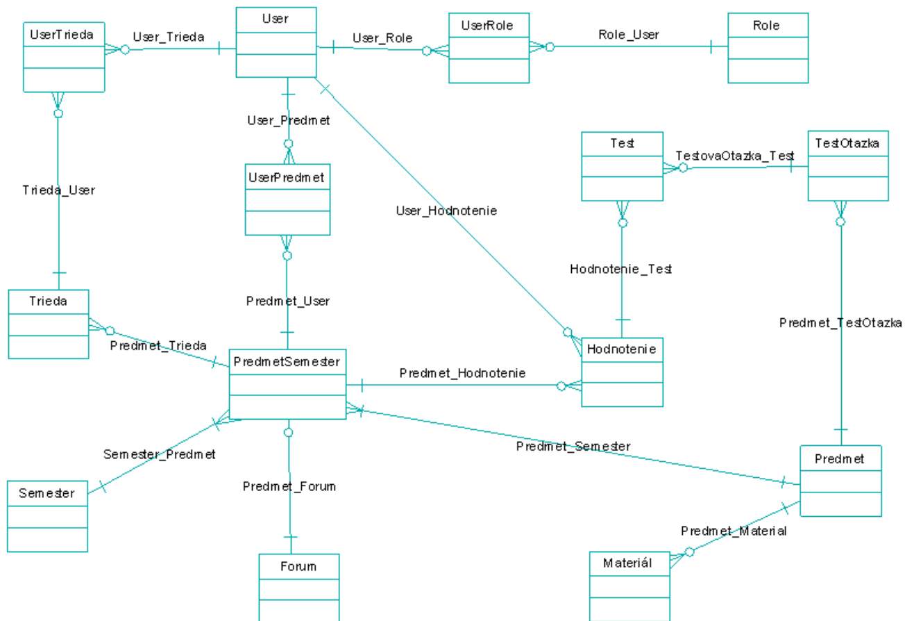
Obr. 8: Logický model údajov
