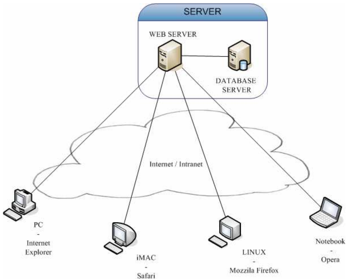
Obr. 36. Architektúra systému.
