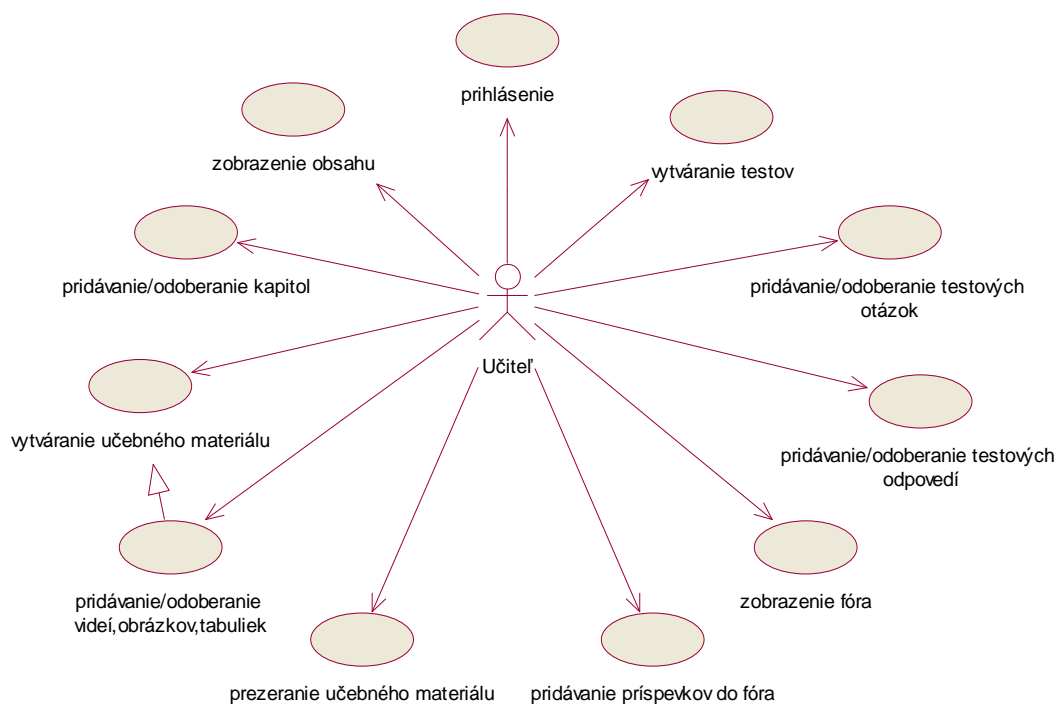
Obr. 30. Diagram prípadov použitia pre učiteľa.
