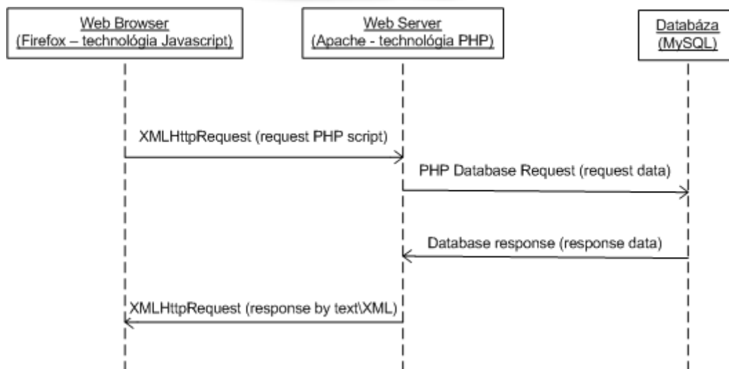
Obr. 47 Diagram komunikácie prototypu s databázou
