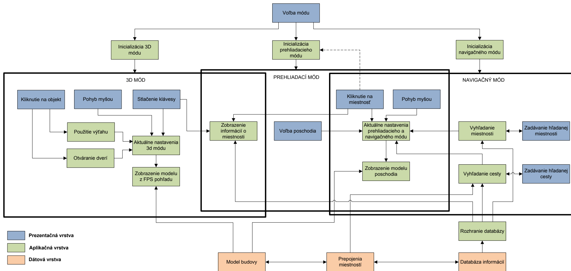
Obr. 32 Architektúra systému - diagram komponentov
