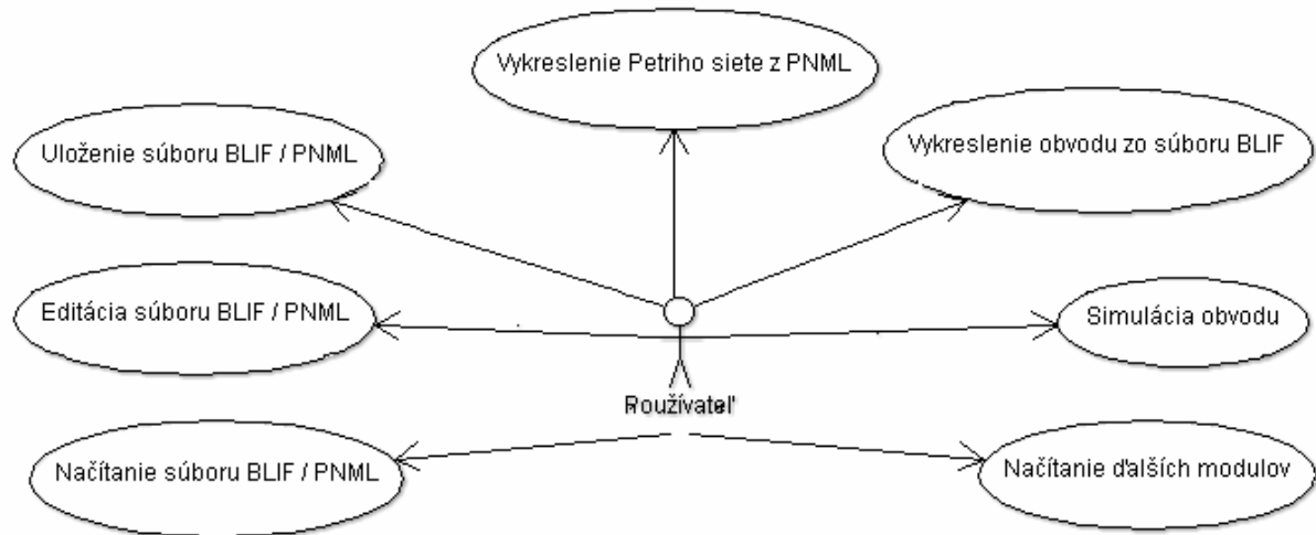
Obr. 2.1: Diagram Prípadov použitia
