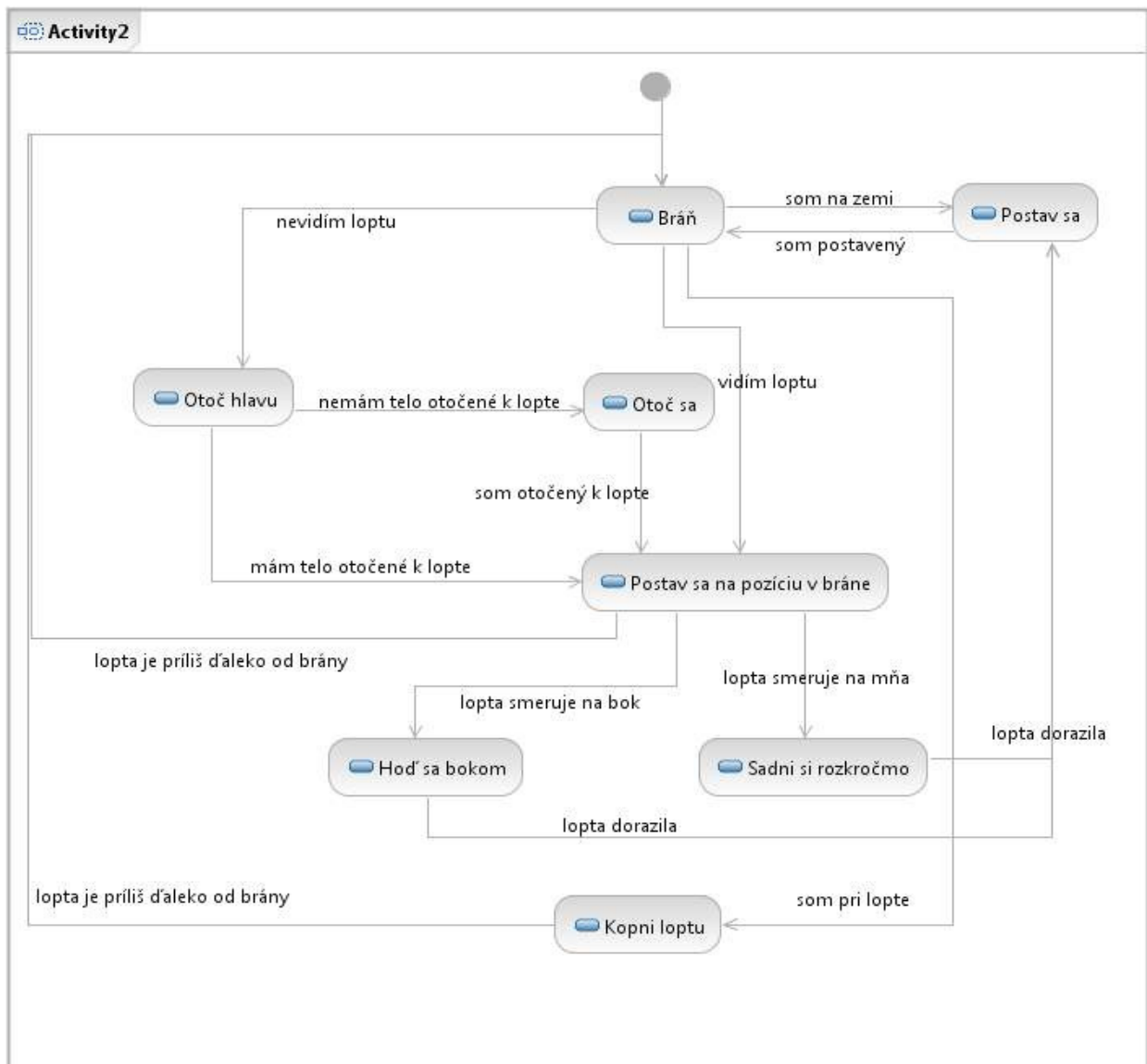
Obr. 54: Rozhodovací strom agenta JIM – bránkar
