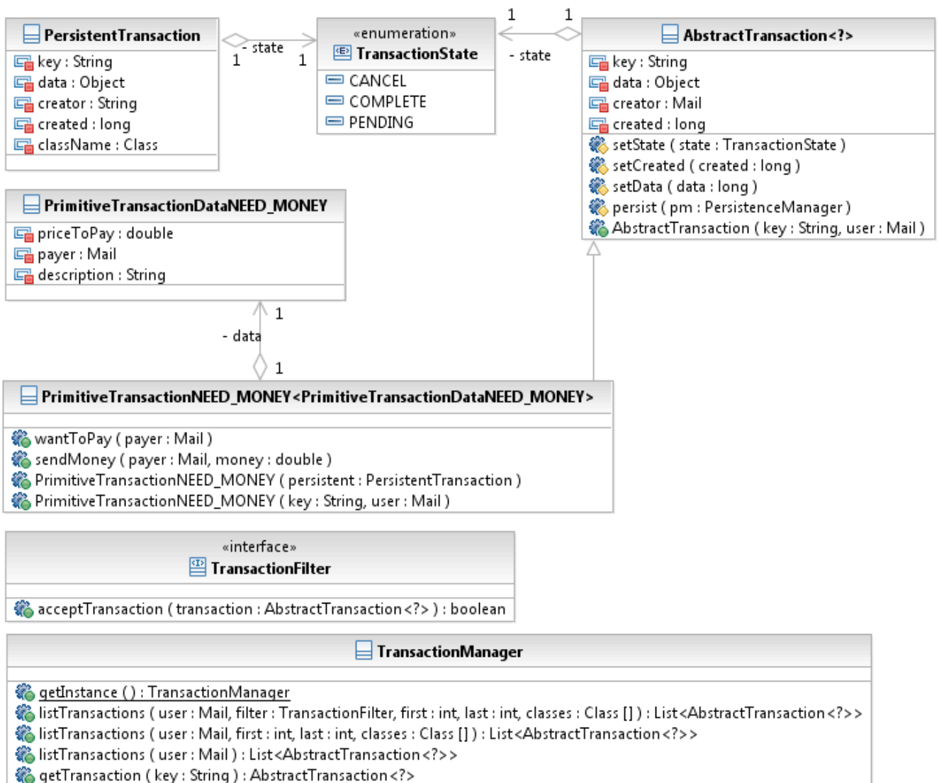
Obrázok 13 Diagram transakcii.
