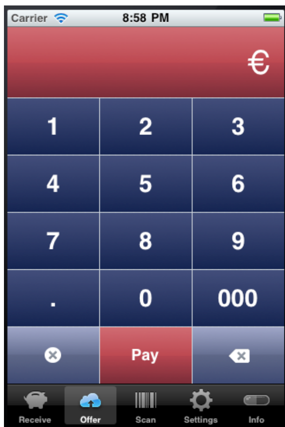
Obrázok 30 Obrazovka Pay
