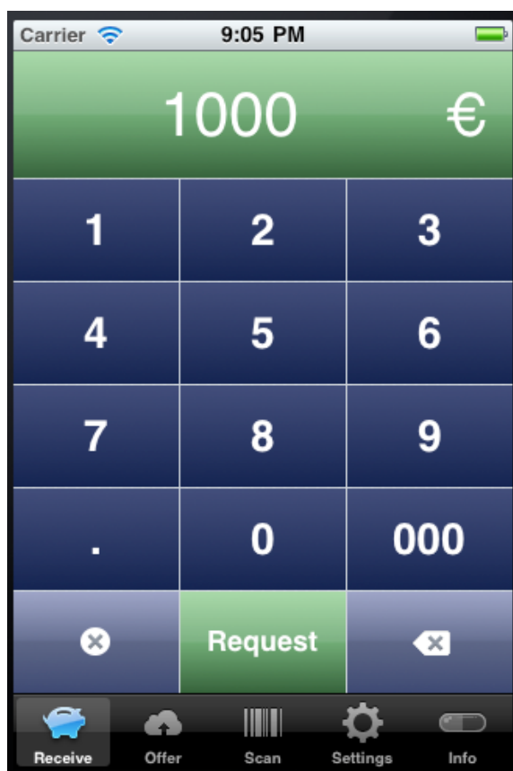
Obrázok 29 Obrazovka Receive
