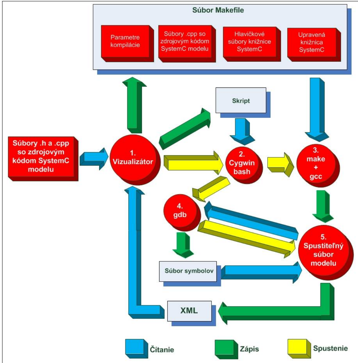
Obr. 7.6: Postup extrahovania informácií.
