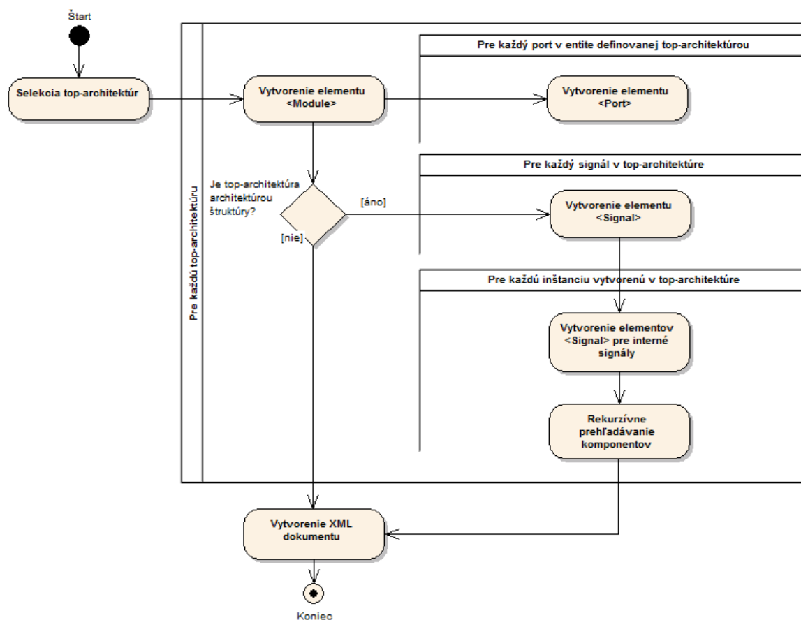
Obr. 7.2: Diagram činností funkcie generujúcej XML súbor
