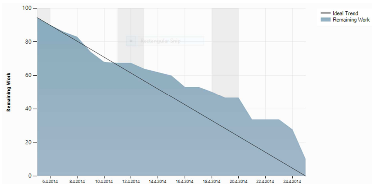
Obrázok 21 - Burndown graf šprintu Iron Maiden
