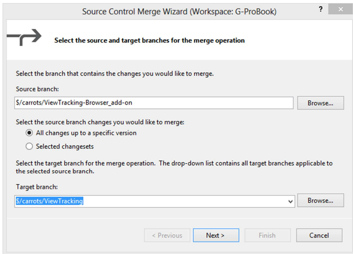
Obrázok 30 - Dialóg pre spájanie vetvy
