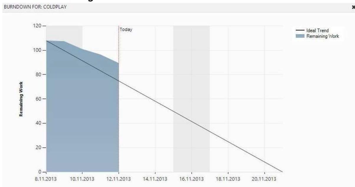
Obrázok 12 - burndown graf
