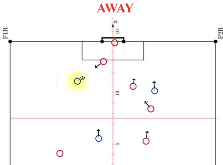
Obrázok 5.3 vzorová situácia 2 útočníka v oktante 4L
