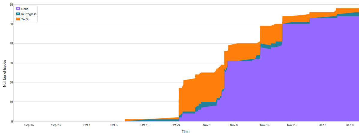
Obrázok 9.2 Cumulative flow diagram po 5. šprintoch
