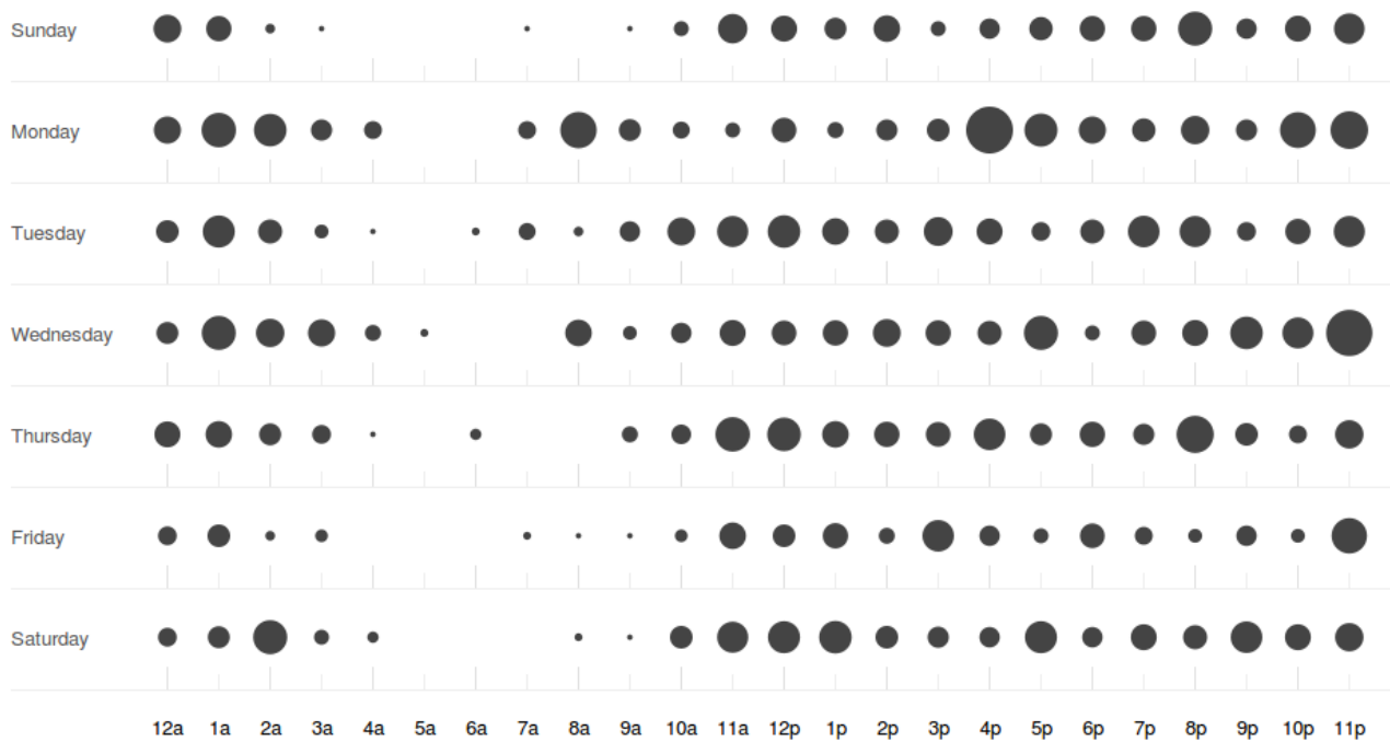
Obr. 5-6: Frekvencia odovzdaní podľa hodín pre repozitár askalot
