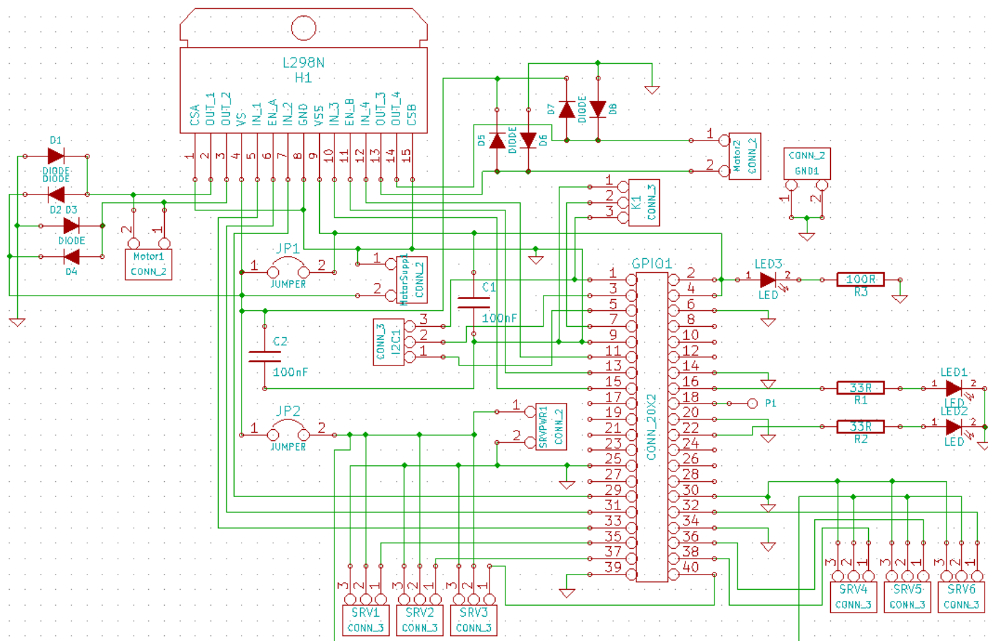
Obrázok 19: Schéma ovládača
