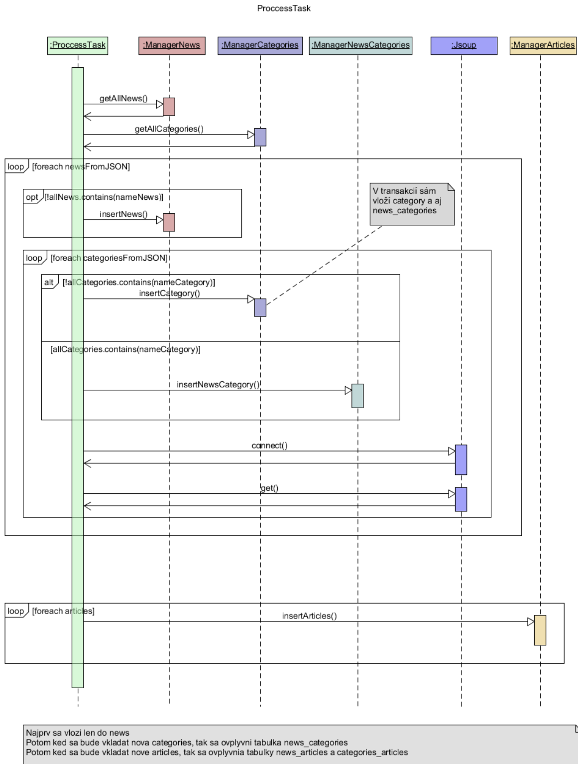
Obr. 21 - Sekvenčný diagram vnútorných činností Loadera
