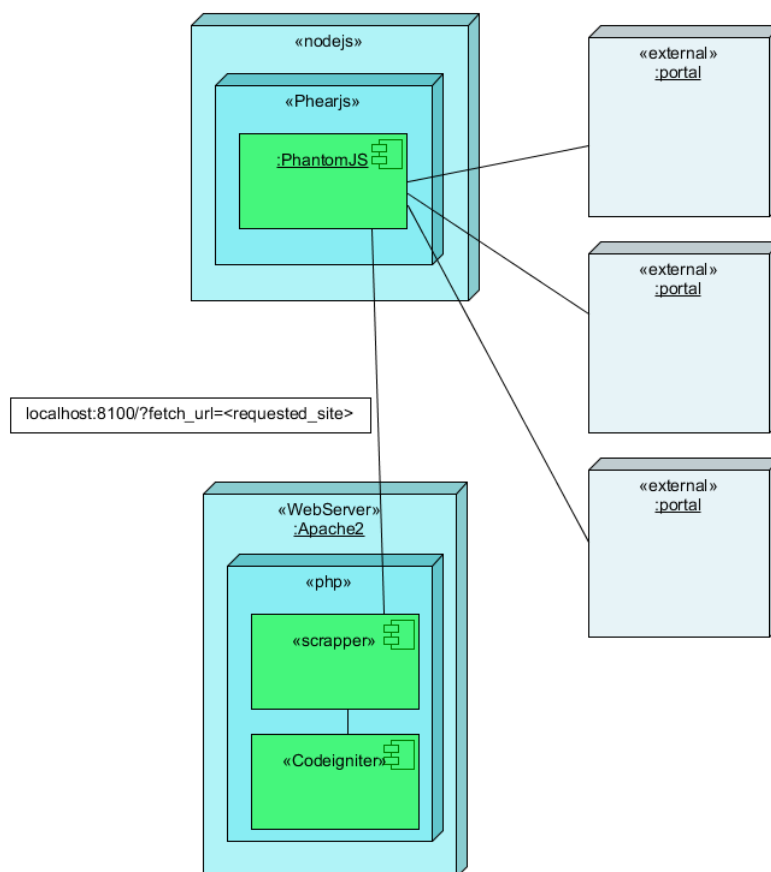
Obr. 27 – Backend architektúra
