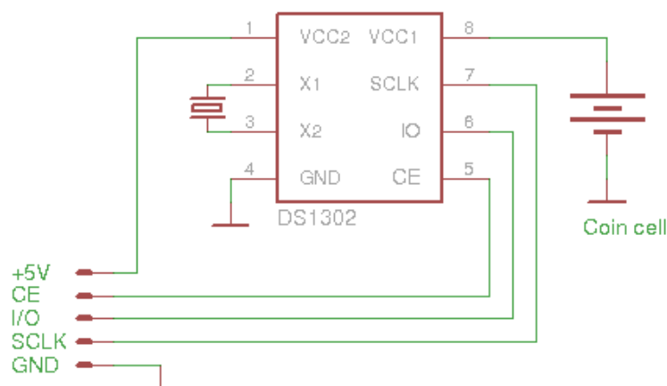
Obrázok 11 Schéma zapojenia RTC modulu [17]
