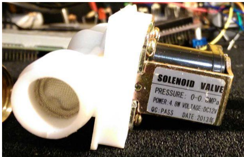
Obrázok 14 Vypúšťací ventil
