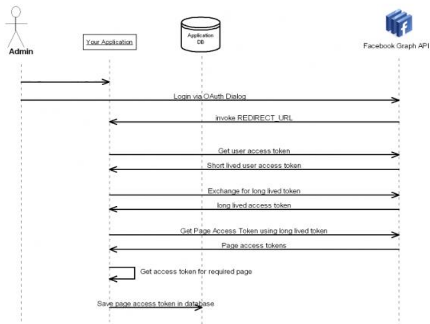
Obrázok 23 Diagram znázorňujúci interakciu medzi adminom, aplikáciou a Facebook Graph API.
