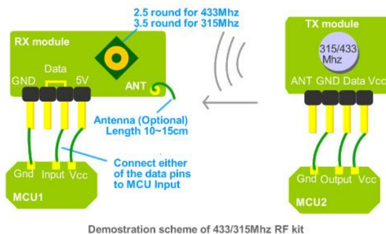
Obrázok 22 Schéma RF transmitting module 433Mhz [23]
