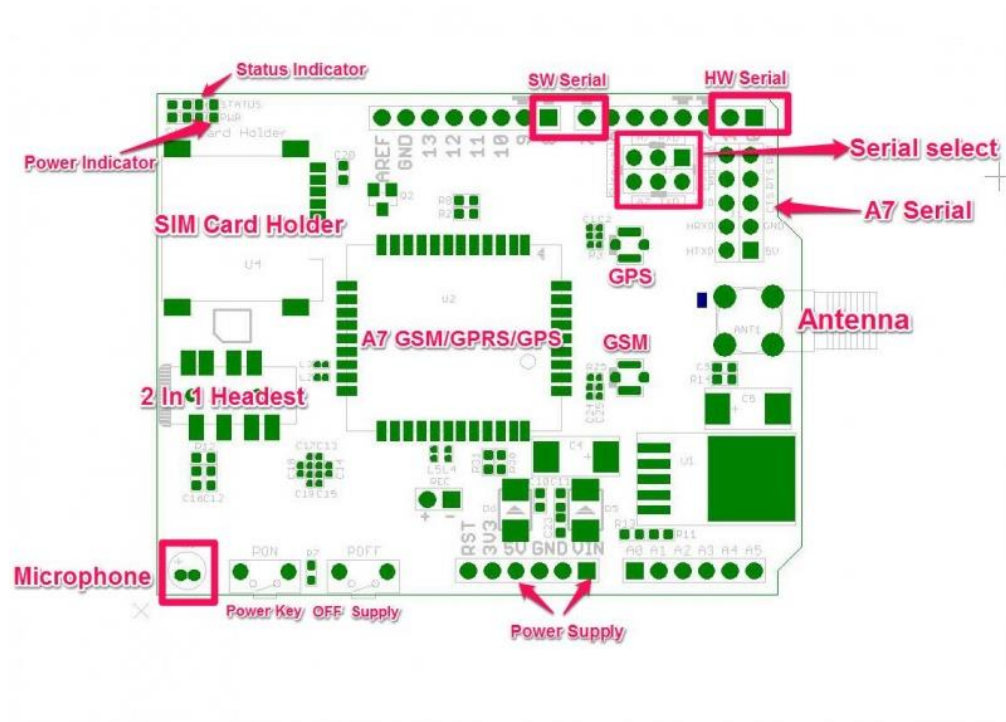
Obrázok 18 Schéma GSM modulu
