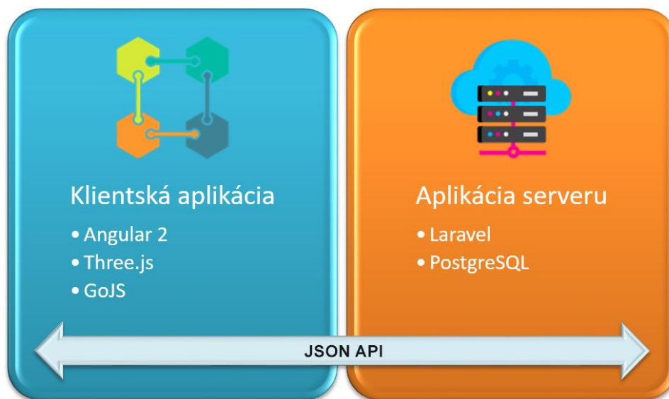
Obrázok: Architektúra aplikácie
